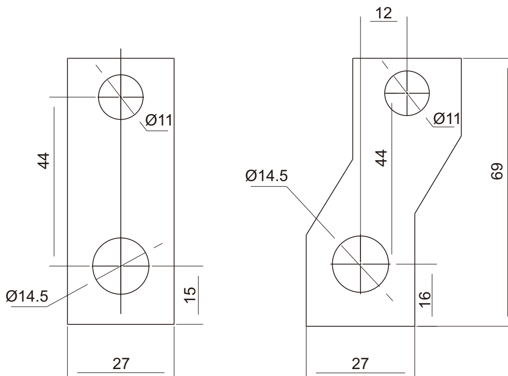
图3 RDM5Z-125附件板
